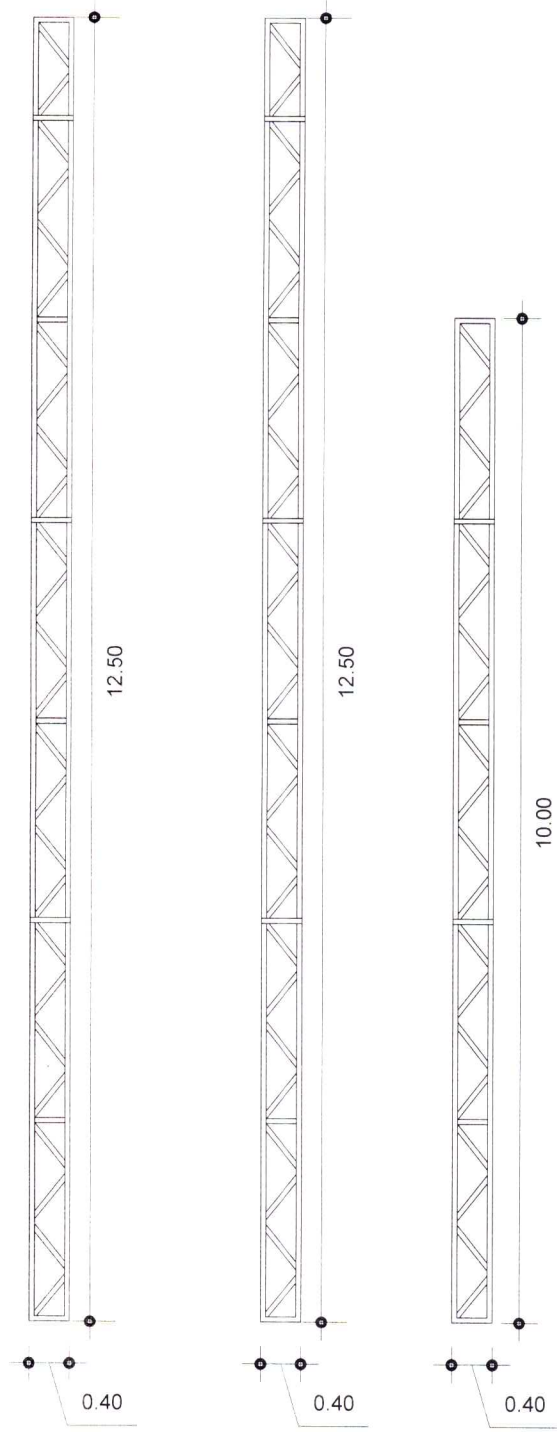
DETALHE DAS TESOURA METALICAS
