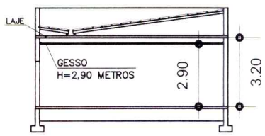
ALTURA DO GESSO SALAS E CORREDOR ESCALA.....1/250
